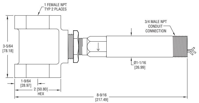
Mit T-Stück
