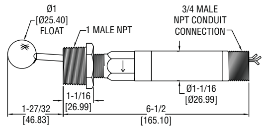
Runder Edelstahlschwimmer
