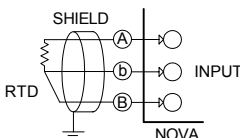
(1) RTD Input
